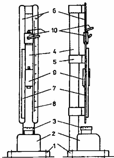
Obr. 1. Schema zkušebního přístroje
