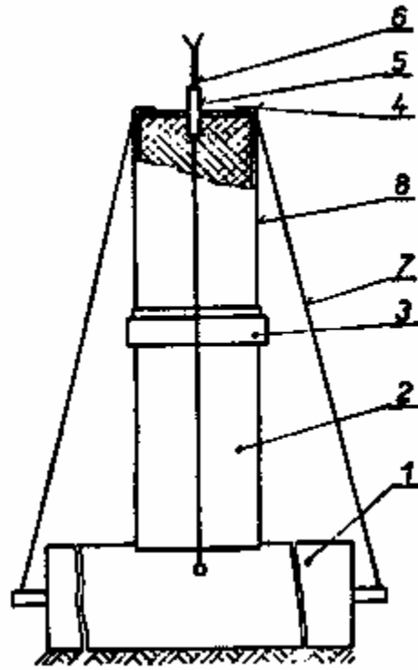
Obr. 2. Zkušební zařízení
