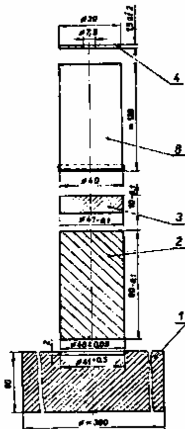
Obr. 1. Zkušební pomůcky
