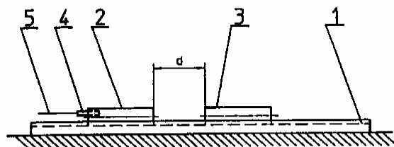
Obr 4. Zkušební zařízení pro metodu B
