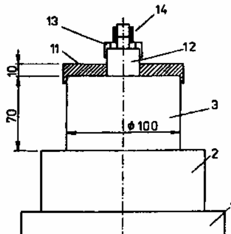
Obr. 4. Sestava zkušební přípravku
