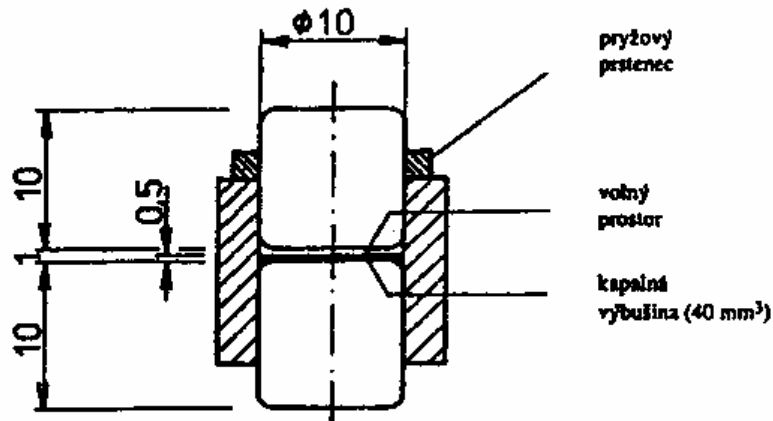
Obr. 5. Úprava pro kapalně trhaviny
