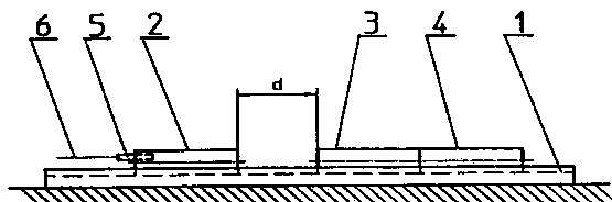
Obr. 1. Zkušební zařízení pro metodu A
