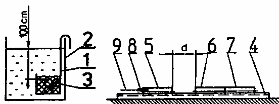
Obr. 5. Zkušební zařízení pro metodu C
