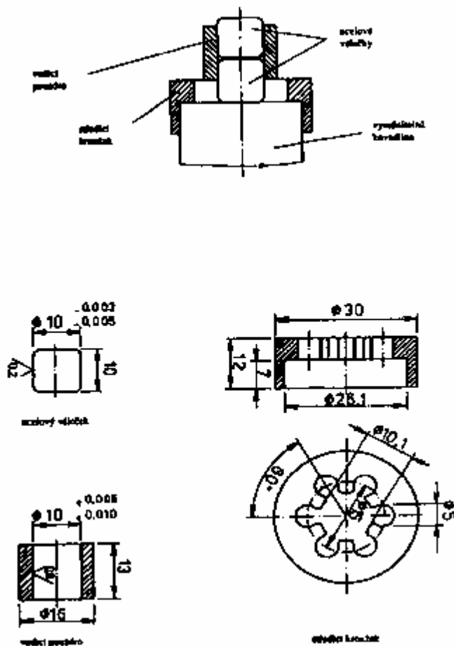
Obr. 3 Zkušební přípravek
