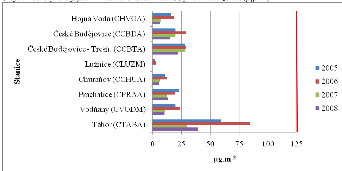
Graf 9. Hodnoty 4. nejvyšší 24-hodinové koncentrace SO 2 – ochrana zdraví (μg.m -3 )
