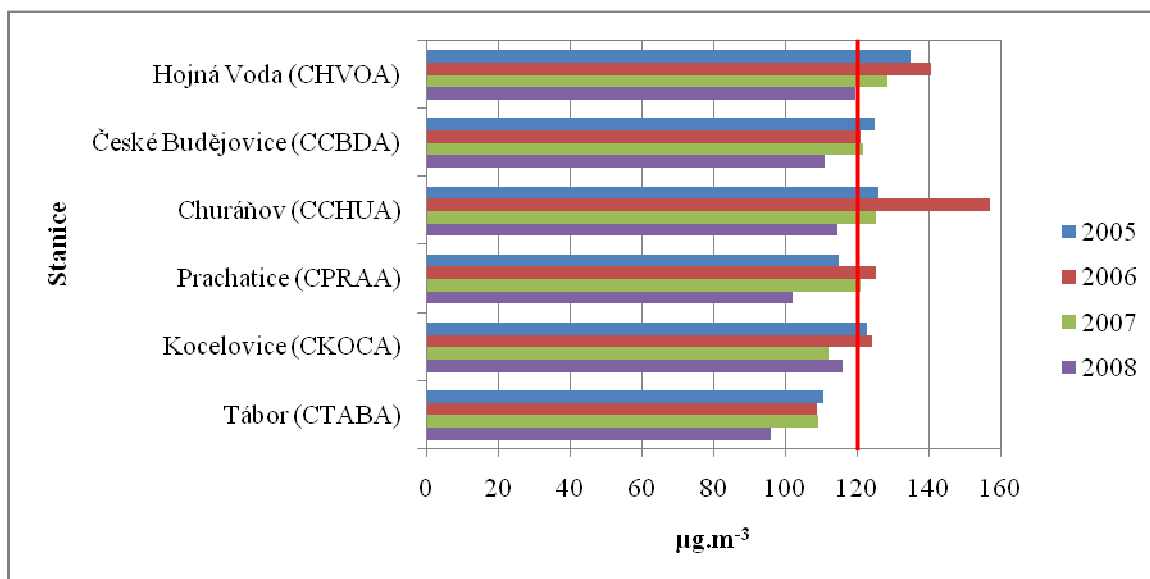
Graf 6. Hodnoty 26. nejvyšší 8-hodinová koncentrace O_3 – ochrana zdraví ( \mu\text{g.m}^{-3} )
