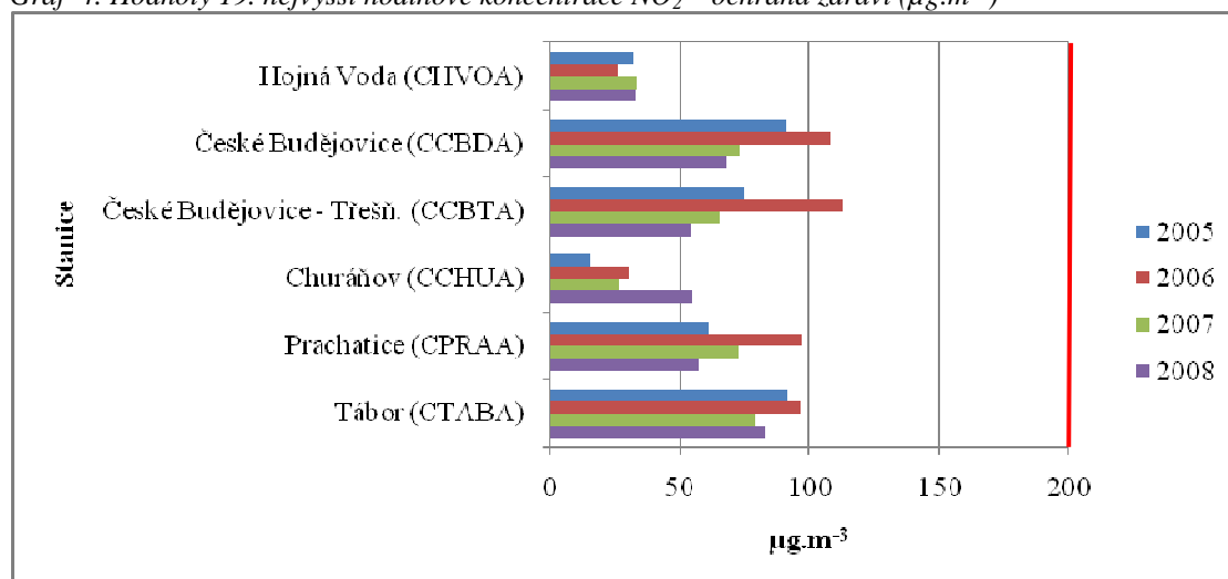
Graf 4. Hodnoty 19. nejvyšší hodinové koncentrace NO 2 – ochrana zdraví (μg.m -3 )
