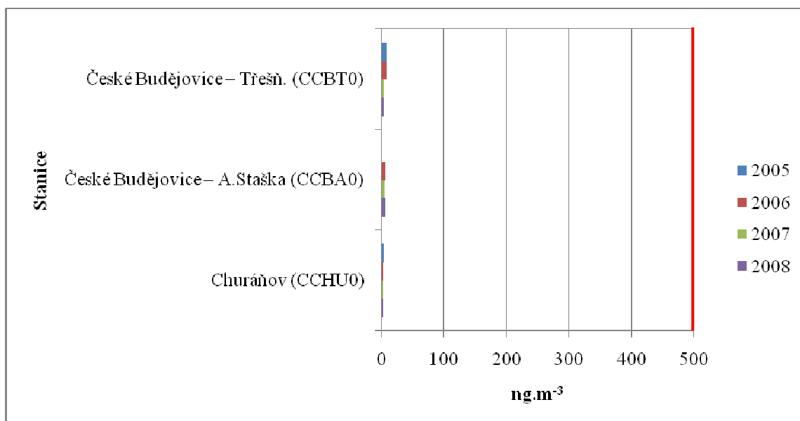
Graf 10. Průměrné roční koncentrace olova – ochrana zdraví (ng.m -3 )
