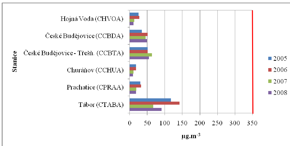
Graf 8. Hodnoty 25. nejvyšší hodinové koncentrace SO 2 – ochrana zdraví (μg.m -3 )
