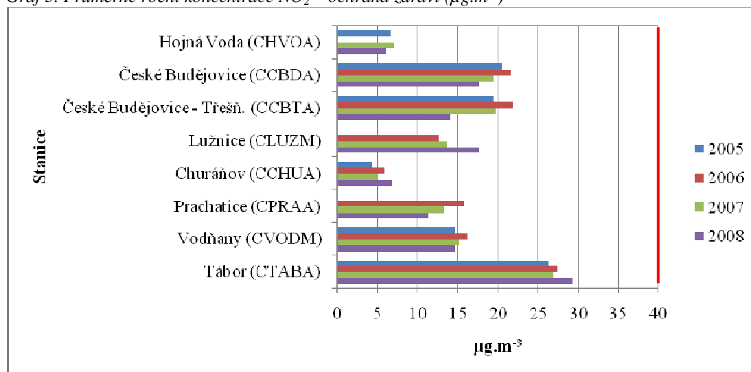
Graf 3. Průměrné roční koncentrace NO 2 – ochrana zdraví (μg.m -3 )
