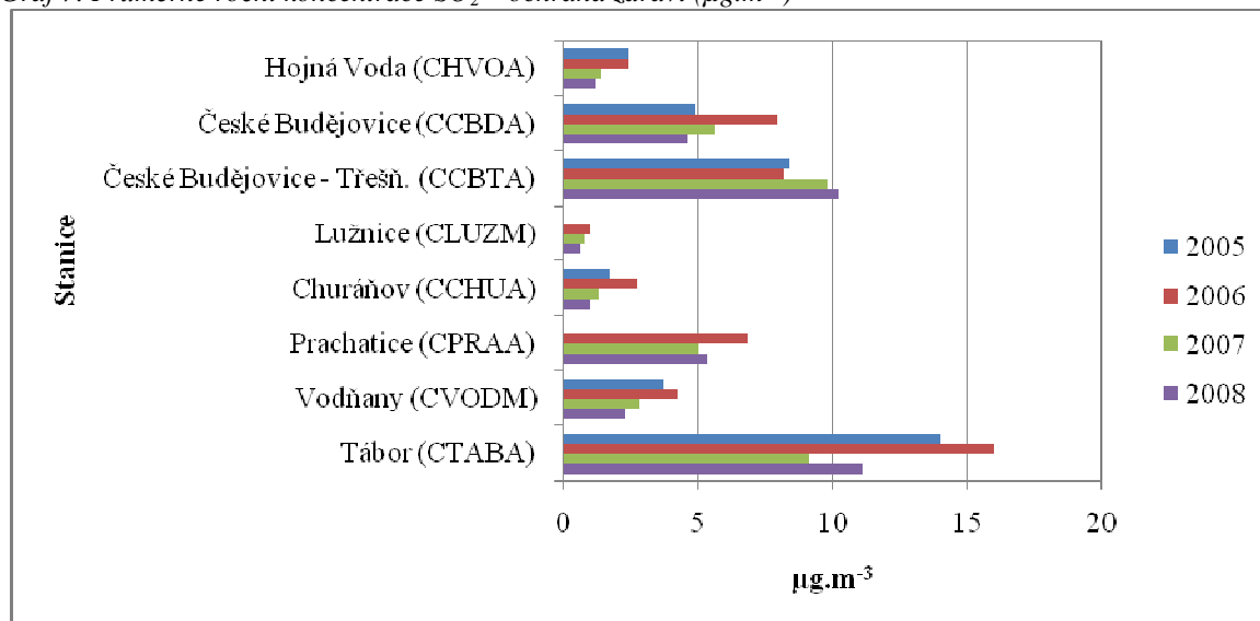
Graf 7. Průměrné roční koncentrace SO_2 – ochrana zdraví ( \mu\text{g}\cdot\text{m}^{-3} )
