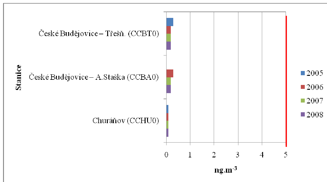
Graf 11. Průměrné roční koncentrace kadmia – ochrana zdraví ( \text{ng.m}^{-3} )
