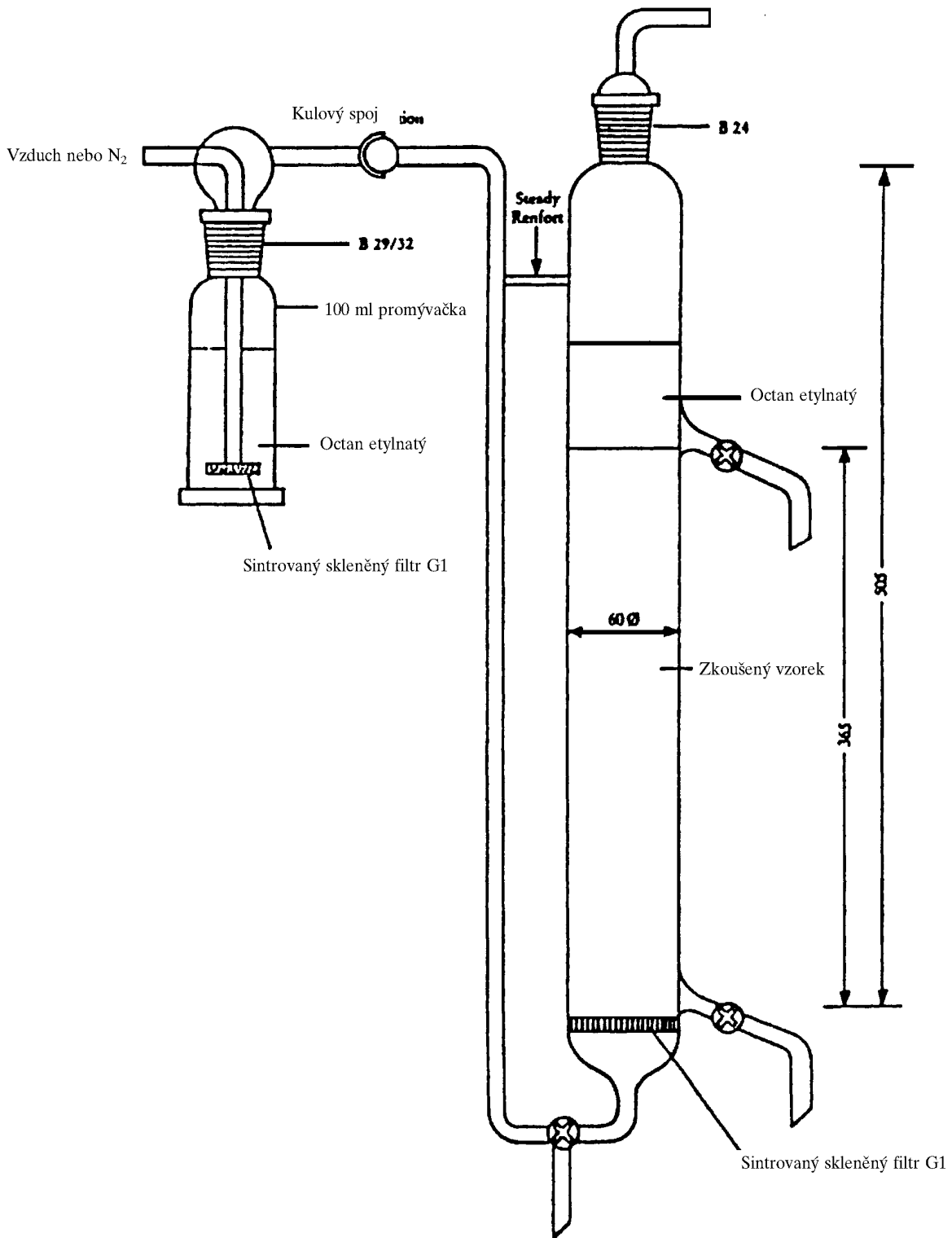
Obrázek 5 Zařízení pro stripování plynem (Rozměry v mm)
