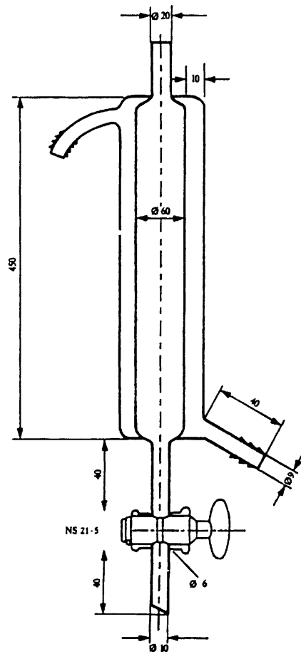
Obrázek 4 Vyhřívaná ionexová kolona (Rozměry v mm)
