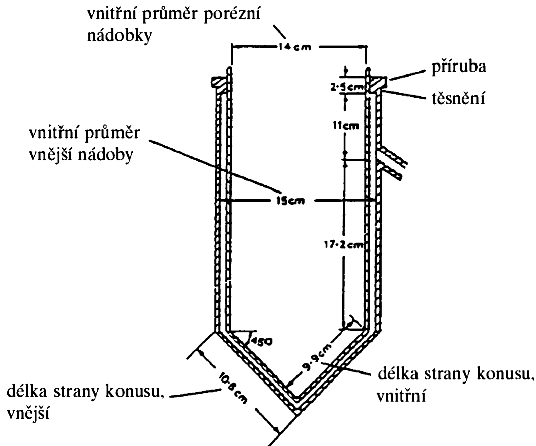
Obrázek 2 Detaily třílitrové vzduchovací porézní nádoby
