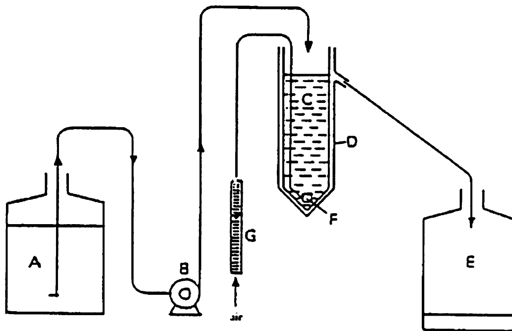
Obrázek 1 Zařízení používané pro stanovení biologické rozložitelnosti
